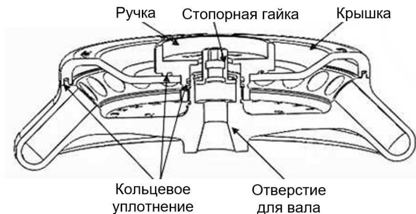
Рисунок 11-1. Ротор, вертикальное сечение
