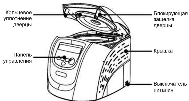
Рисунок 5.1 Вид спереди
