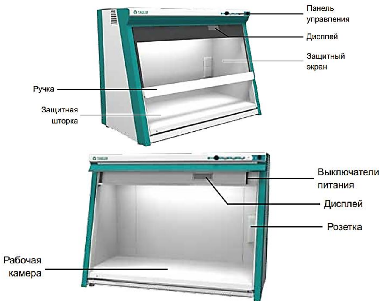
Рисунок 2 – Устройство и основные части бокса (вид спереди)
