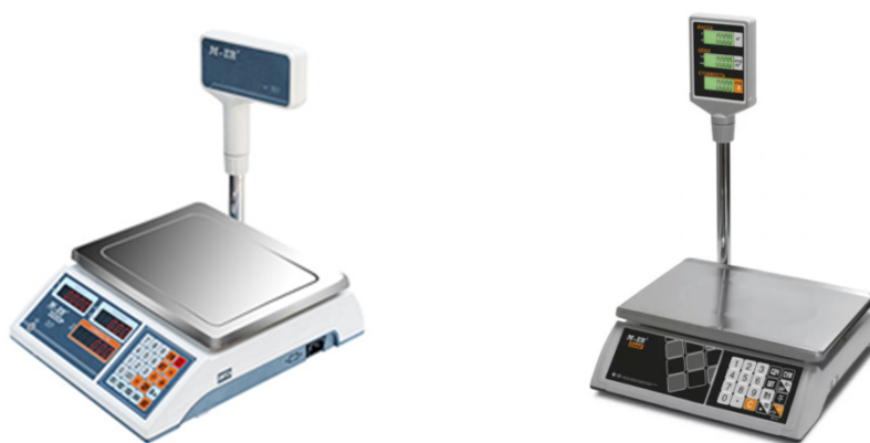
Рисунок 2 — Весы настольного исполнения с вторичным дисплеем на стойке
